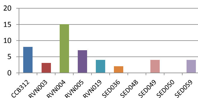
Fig. : activiteitsconcentratie aan radium-226 en cesium-137 in de sedimenten van Waalse waterlopen.
