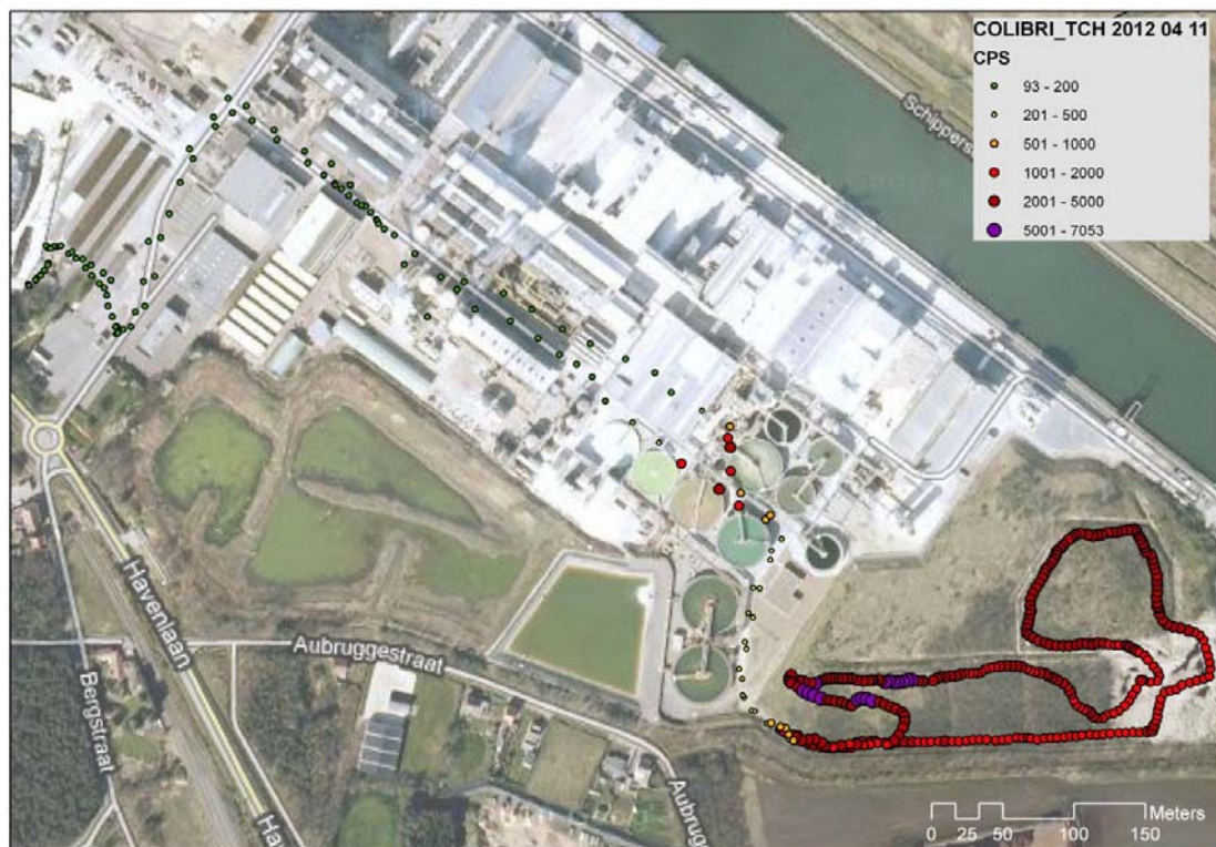
Fig. 2 : mesures de rayonnement gamma (en coups par seconde) à la surface de la décharge située dans le périmètre de l'entreprise de TESSENDERLO CHEMIE à Ham.
