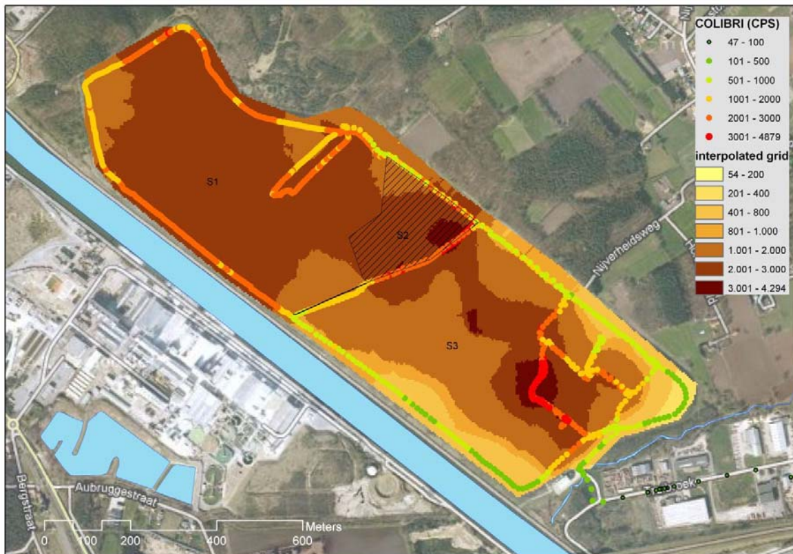
Fig. 1 : mesures de rayonnement externe (en coups par seconde) sur la mono-décharge Veldhoven de TESSENDERLO CHEMIE
