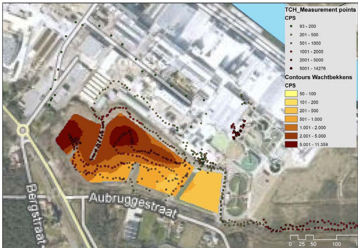
Fig. 3 : mesures de rayonnement gamma (en coups par seconde) à la surface de l'ancien bassin de rétention des eaux usées de l'entreprise de TESSENDERLO CHEMIE à Ham.
