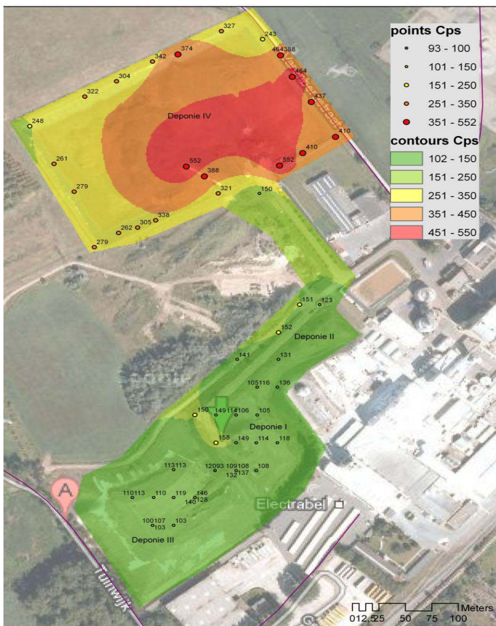
Fig. 4 : mesures de rayonnement gamma (en coups par seconde) à la surface de des décharges de KRONOS EUROPE à Gand.
